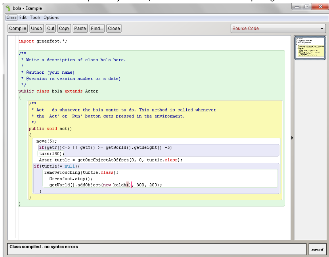
Gambar 57 method jika kalah
