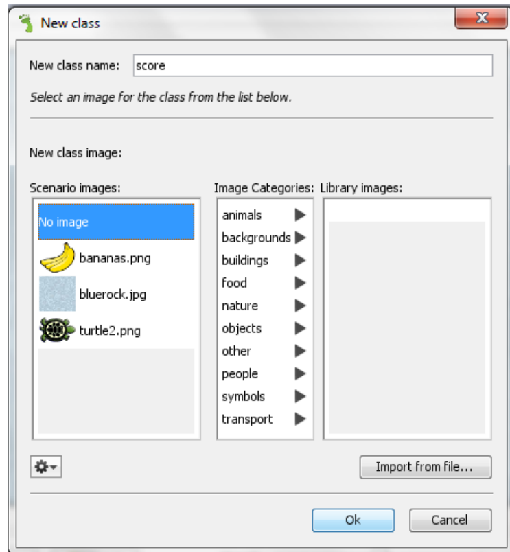
Gambar 48 membuat score
