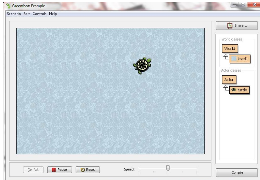
Gambar 45 object bergerak
