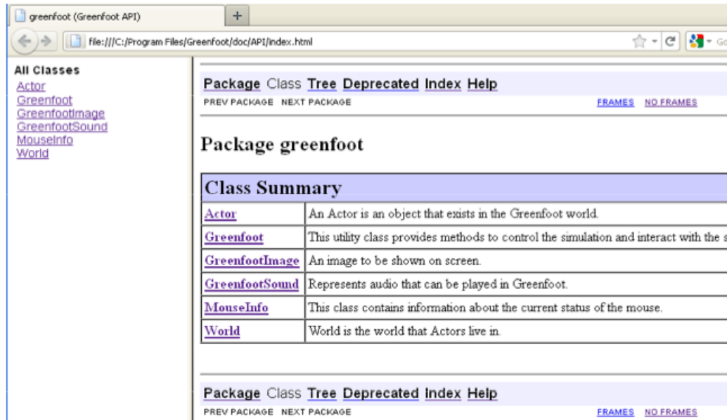
Gambar 32 API
