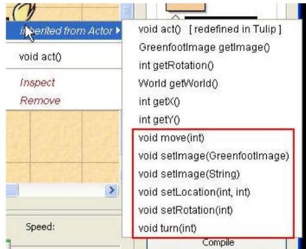
Gambar 9 Method dengan return type Void
