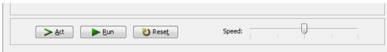
Gambar 1 Kontrol Eksekusi
