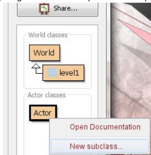
Gambar 39 menambahkan actor
